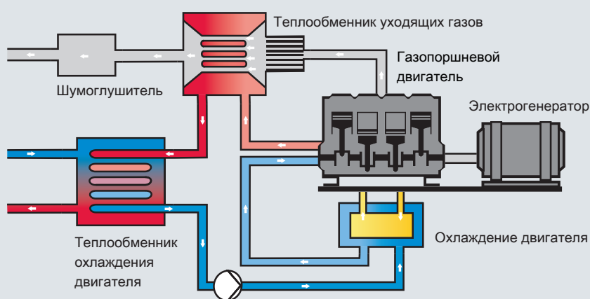
Рис. 2. Функциональная схема когенерационной установки
